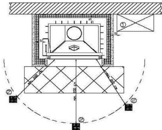
Abb. 1.5. Mindestabstand von Gegenständen der Innenraumausstattung
