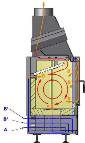
Abb. 1.7. Luftumwälzung: A-Luft unter den Rost B1-Sekundärluft, B2-Luftvorhang
