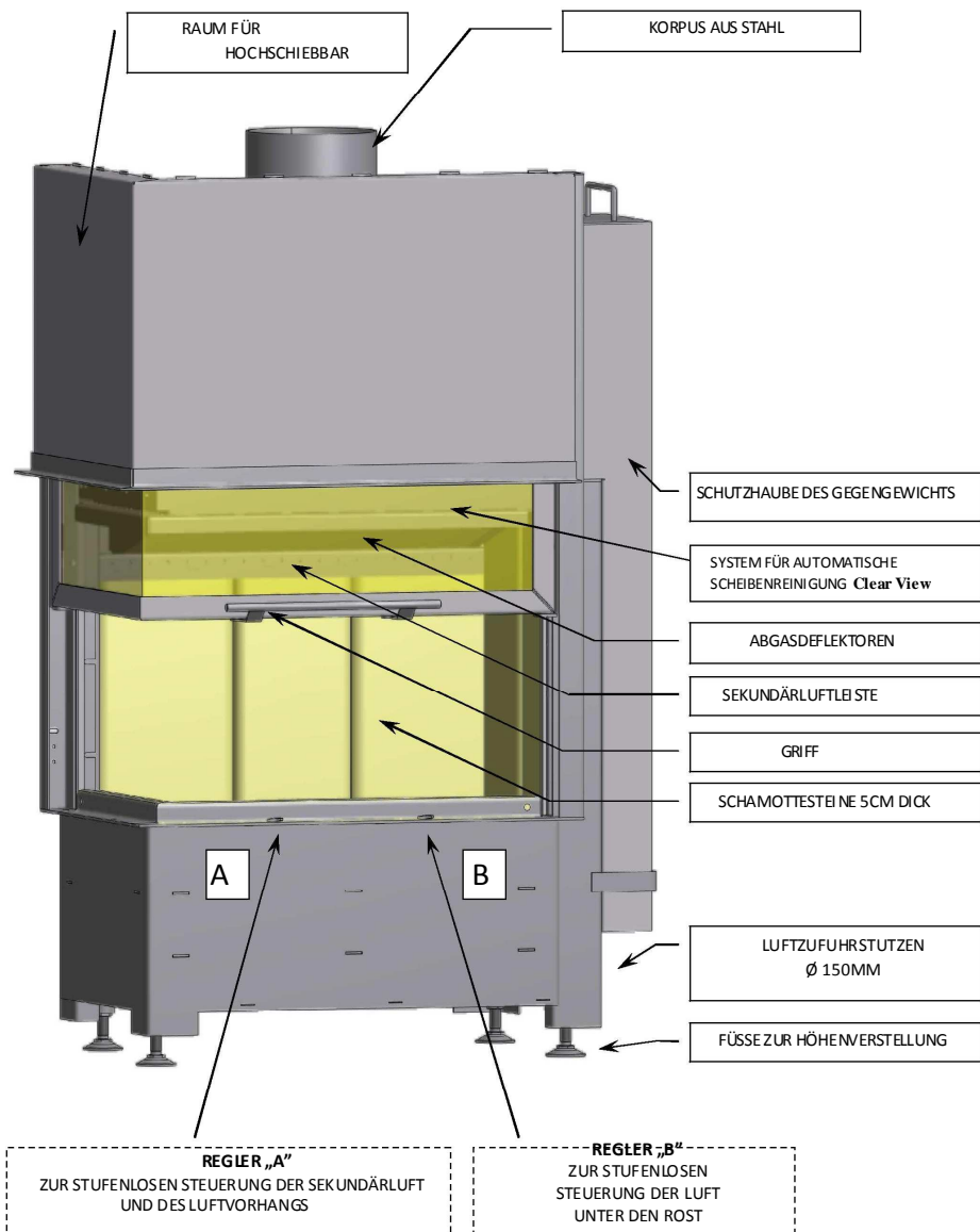
Abb. 1.1. b Aufbau eines exemplarischen Volcano 2Lh-Einsatzes
