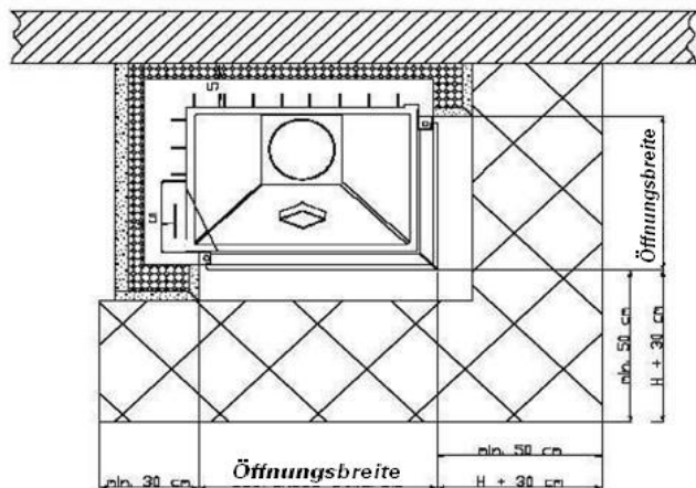
Abb. 1.4. Die Mindestgröße der Schutzunterlage.
